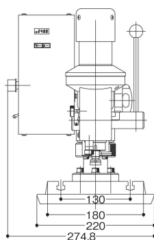
BDM-660 テーブルT溝部分寸法図
