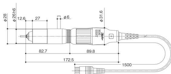
φ3 コレットチャック (CP30H) 装着
