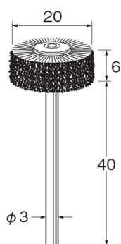
鉄波線 線径φ0.15
