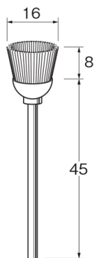
ステンレス線 線径φ0.1
