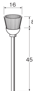
鉄波線 線径φ0.15
