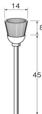
ナイロン 線径φ0.2
