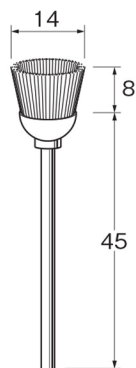
タンピコ (植物繊維)
