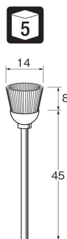
軸付カップ型ブラシ
