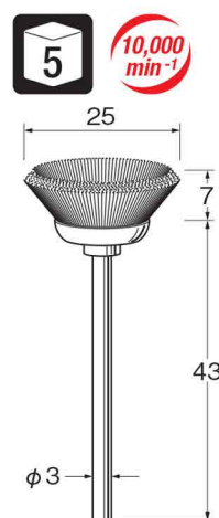
軸付ベベル型ブラシ
