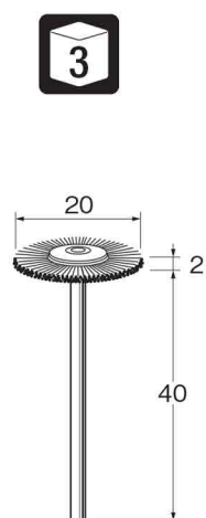
軸付ホイール型ブラシ
