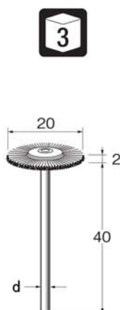
軸付ホイール型ブラシ
